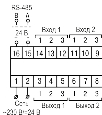
Рисунок 5.5 – Общая схема подключения ТРМ12–Щ5
