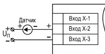
Рисунок 5.21 – Схема подключения пассивного датчика с токовым выходом 0...5 мА или (4)...20 мА
