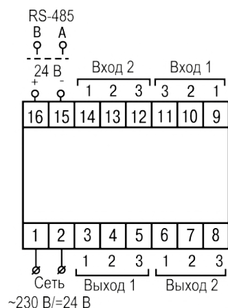
Рисунок 5.6 – Общая схема подключения ТРМ12–Д
