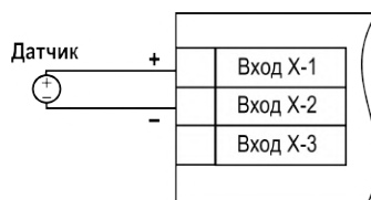
Рисунок 5.20 – Схема подключения активного датчика с выходом в виде напряжения 0...5 В и 0...10 В
